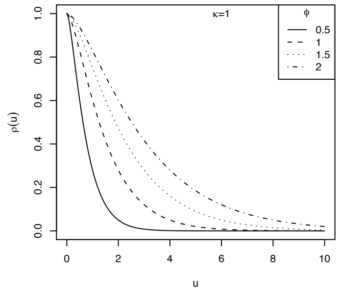
Matern-Familie
