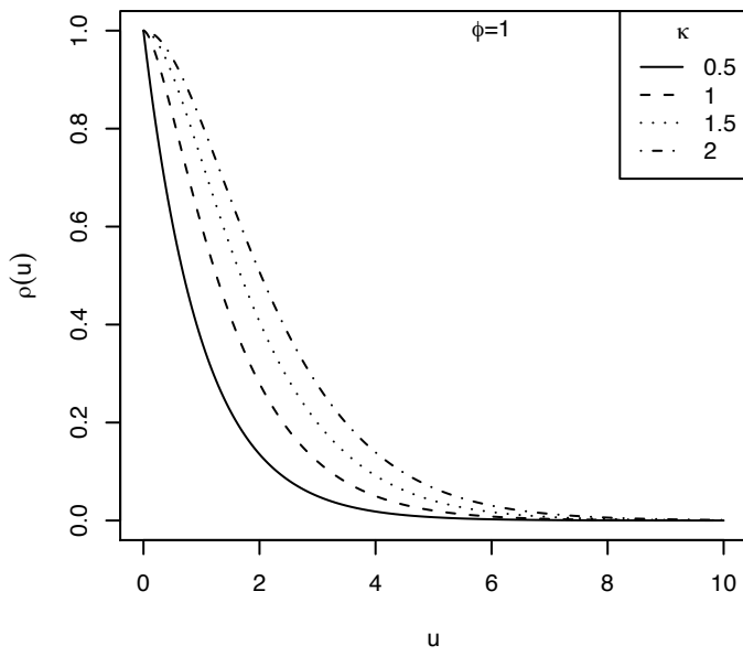
Matern-Familie
