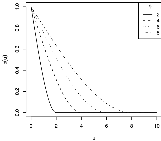
Sphaerische Familie
