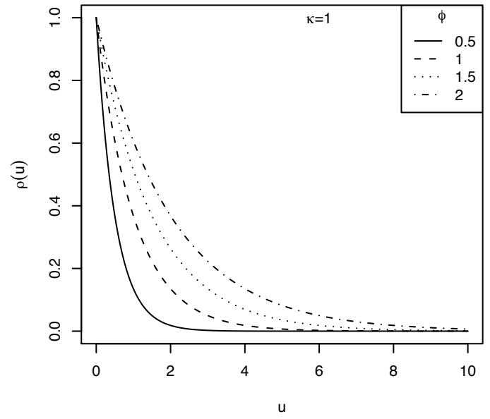
Potenz-Exponentialfamilie
