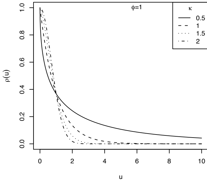
Potenz-Exponentialfamilie
